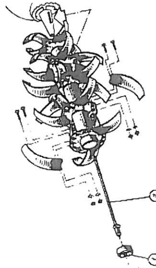
1 – nakrętka zabezpieczająca 2 – pręt ściągający Rys. 5. Dokręcanie prawego bębna roboczego
